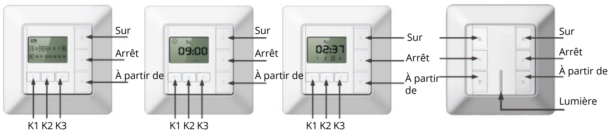
Émetteur mural radio 16 canaux RE 203-16C
