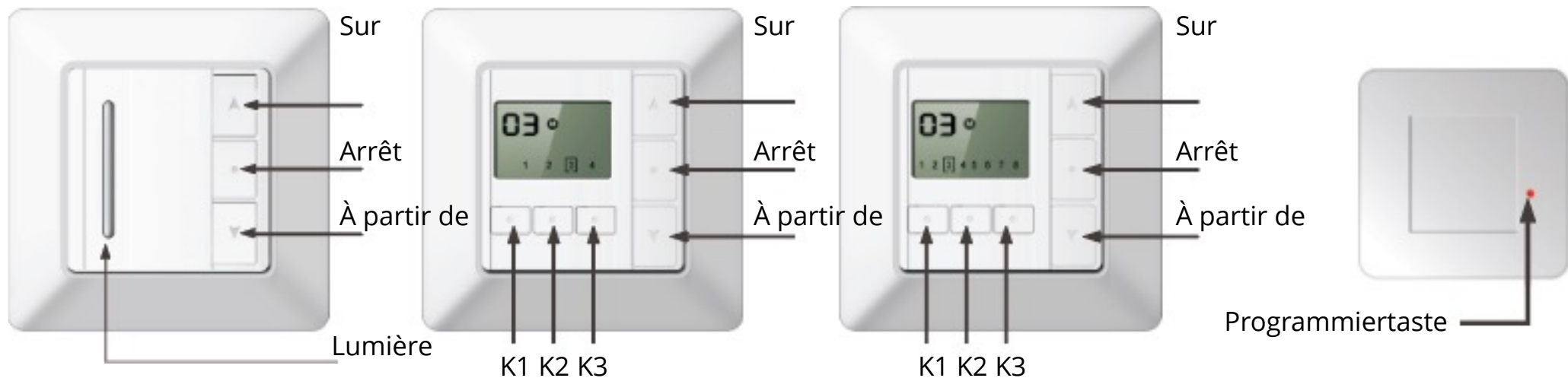
Émetteur mural radio monocanal RE 201
